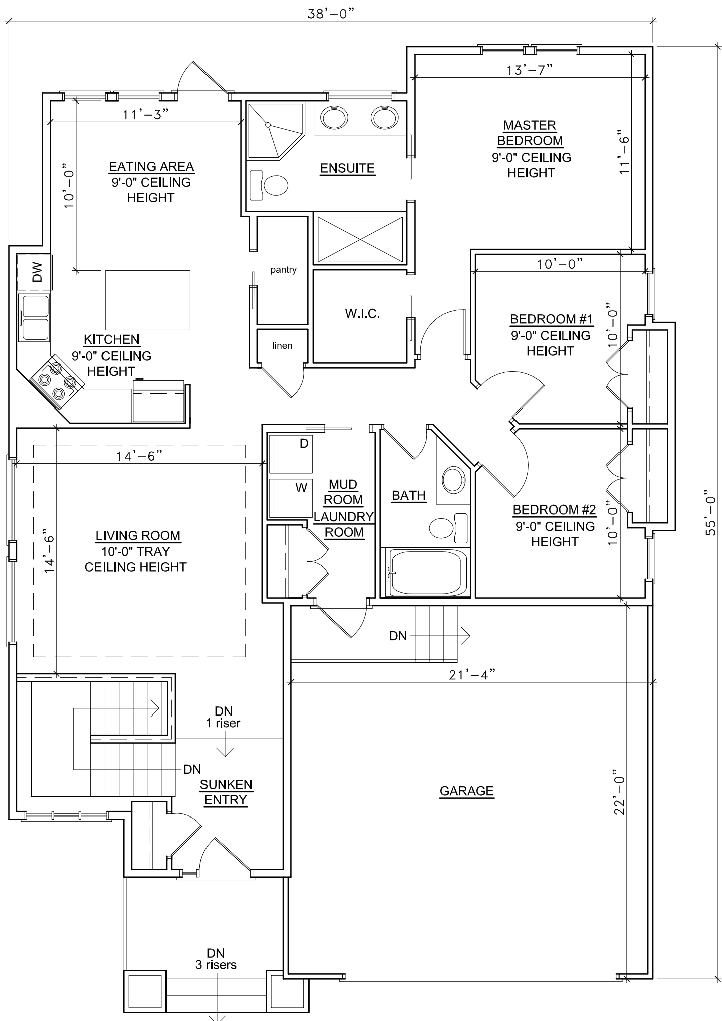
M A I N F L O O R P L A N
